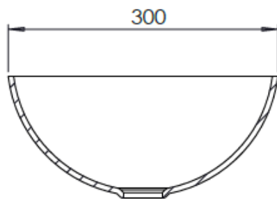
SEZIONE B-B
