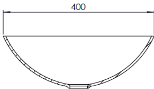
SEZIONE A-A
